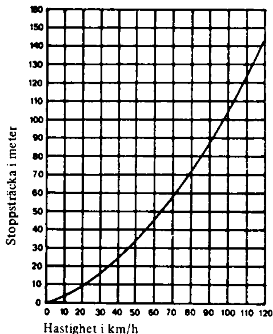
Sambandet mellan hastighet och stoppsträcka.
