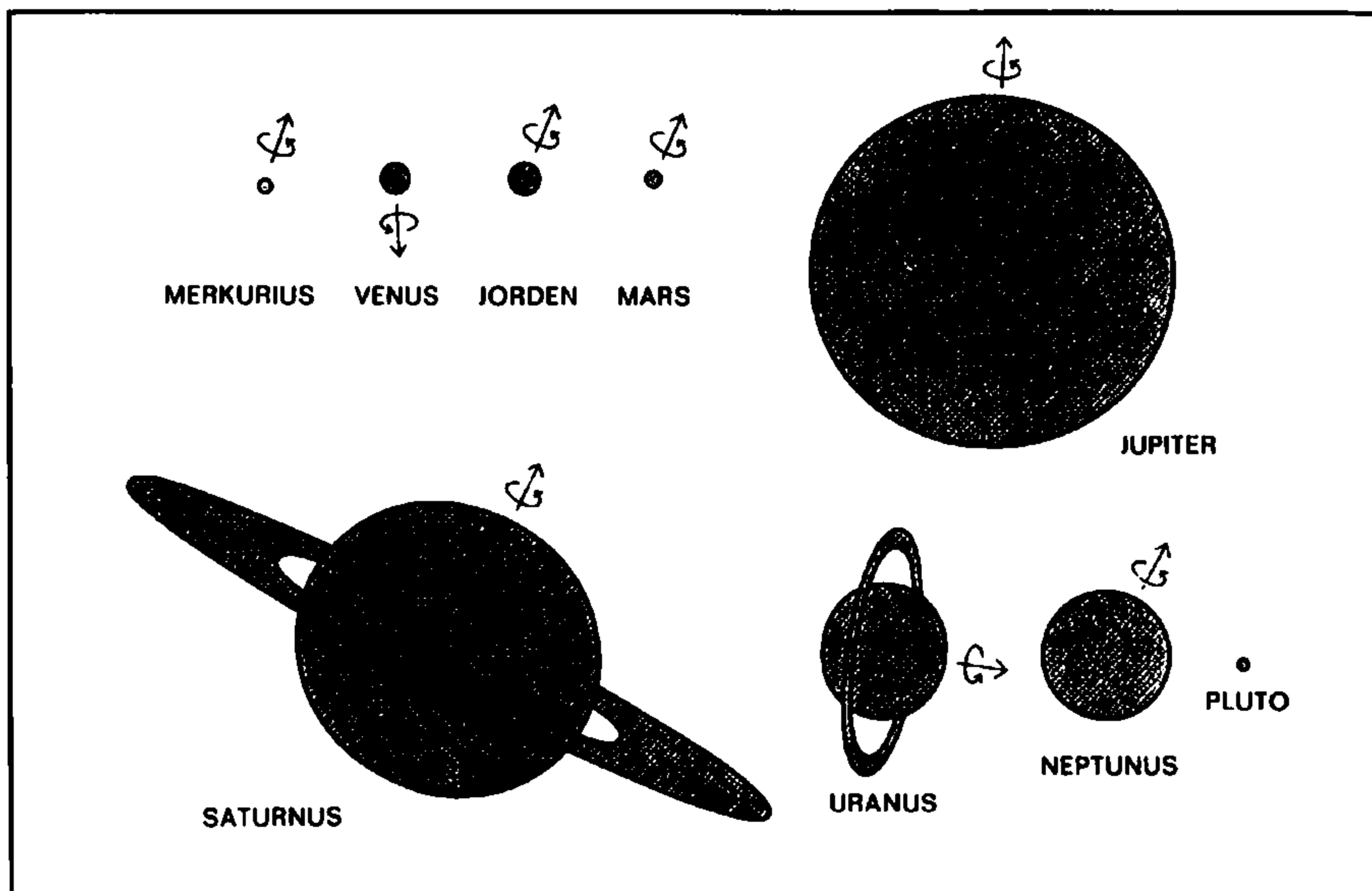
Rotationsaxlarnas riktning hos solsystemets huvudplaneter.
