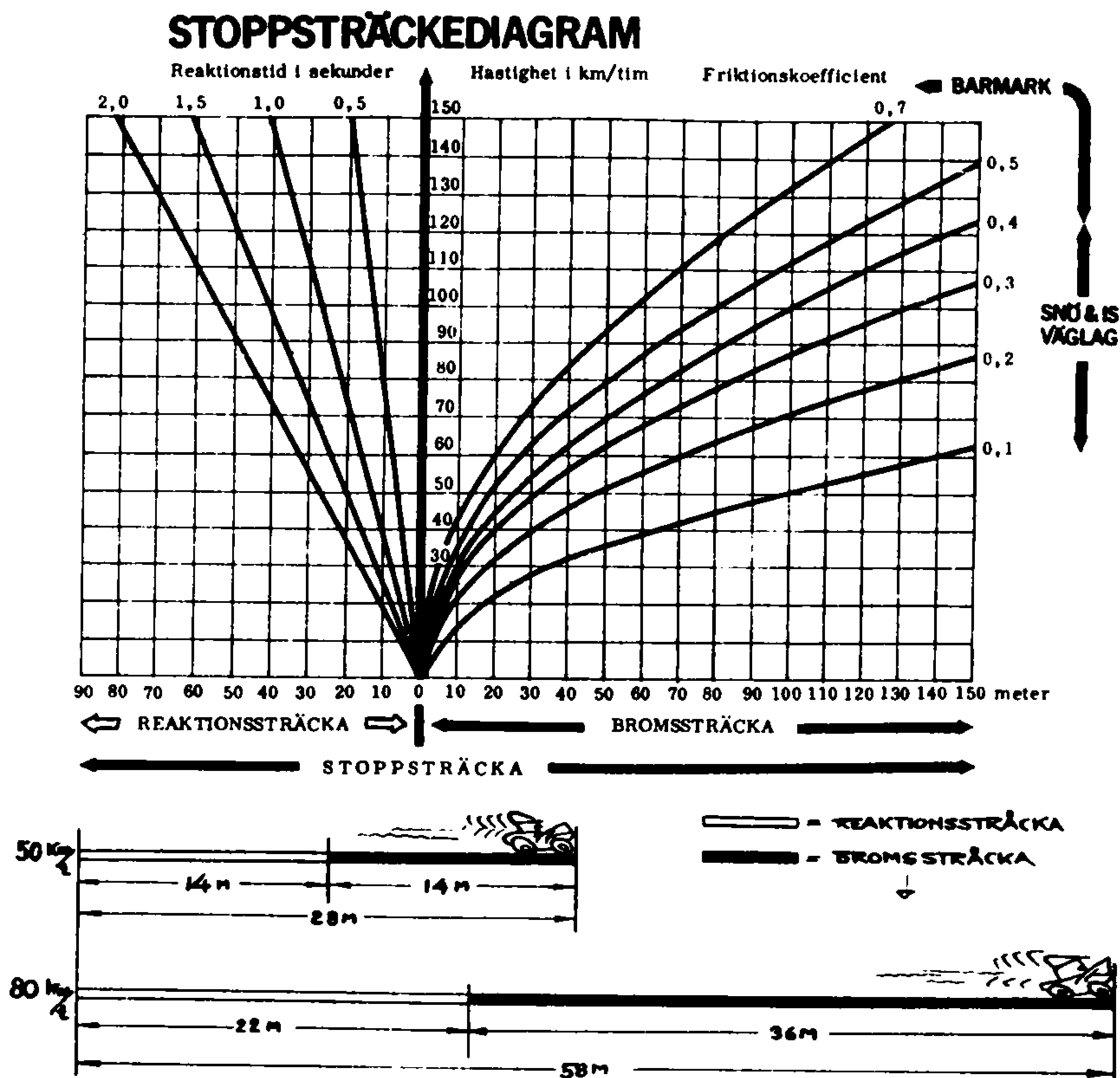
FIGUR 5. STOPPSTRÄCKEDIAGRAM
